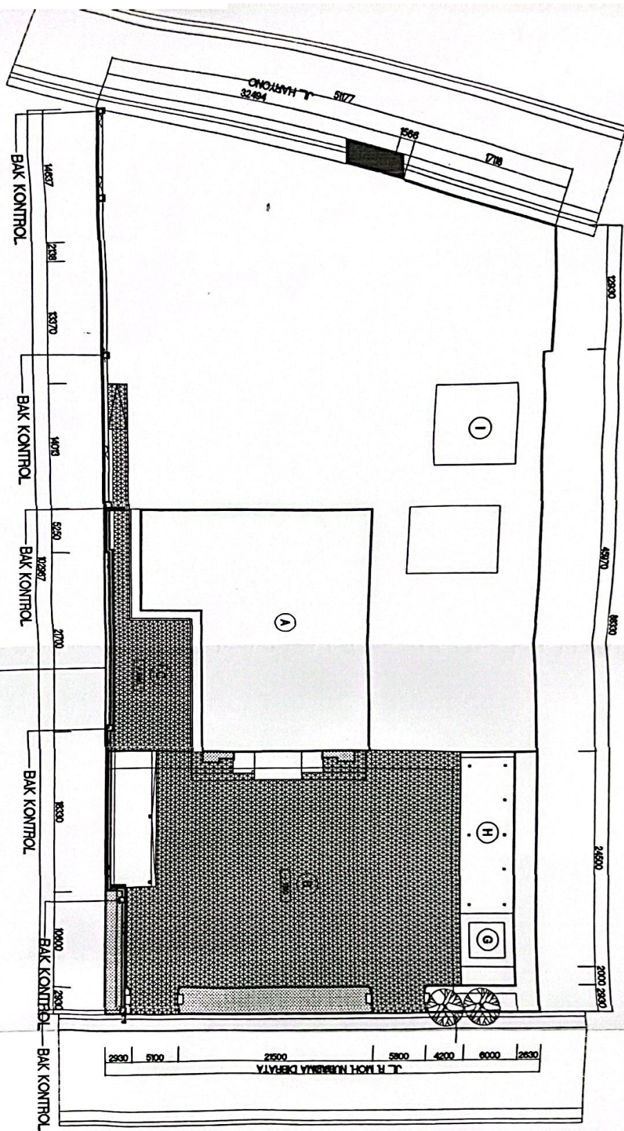
1 SITEPLAN RENCANA DRAINASE 1:400
